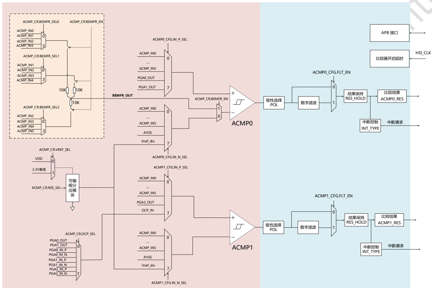
图 22-1 ACMP 结构框图
