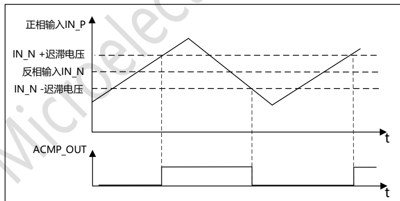
图 22-2 比较器迟滞
