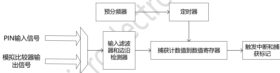
图 11-1 捕获模式
