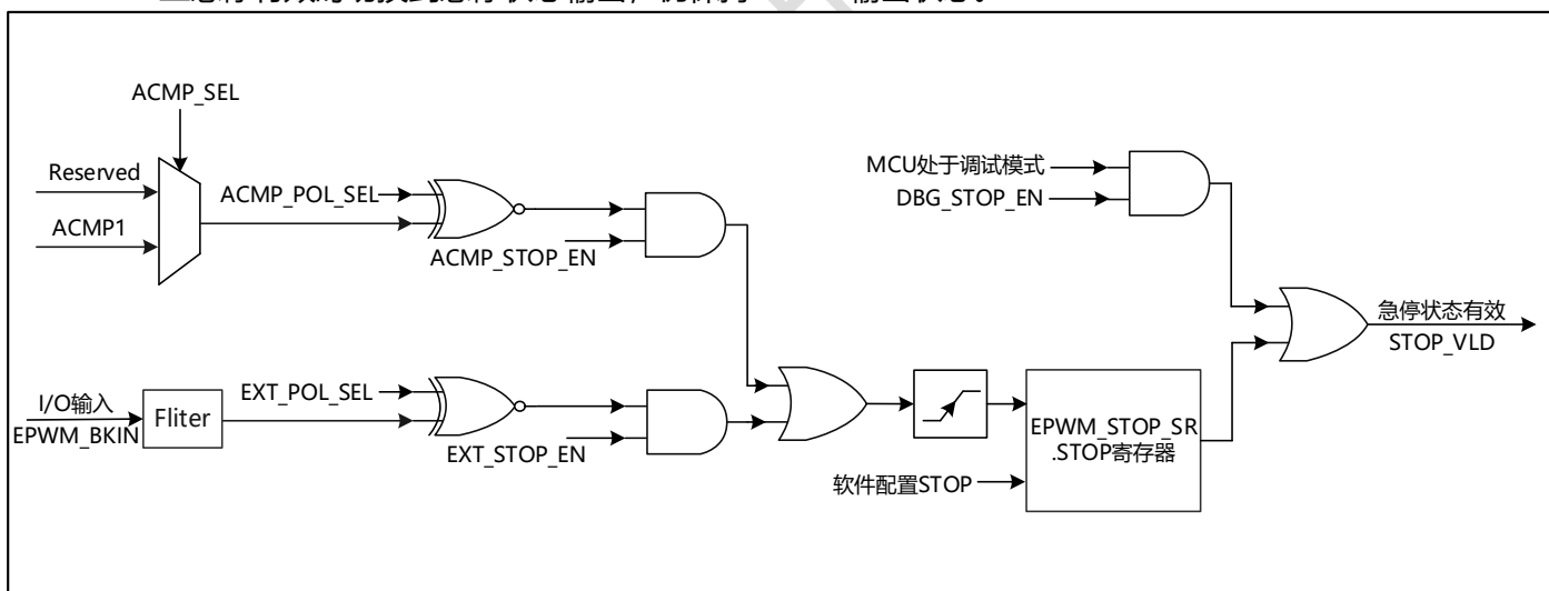
图 11-5 急停控制模块
