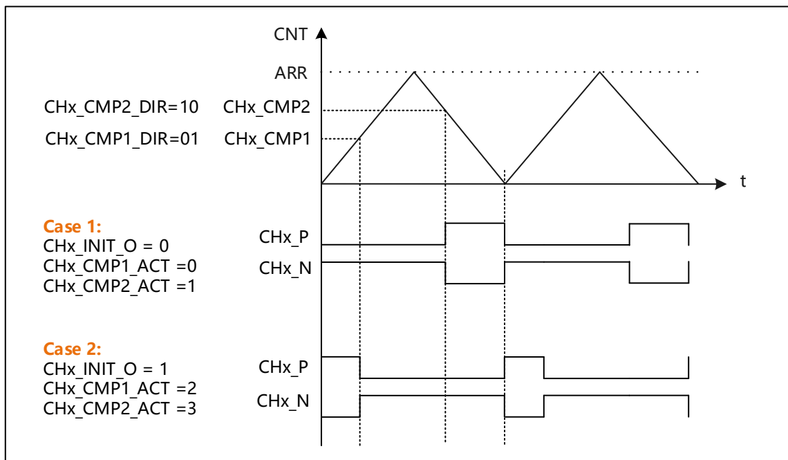
图 11-3 输出互补 PWM 示意
