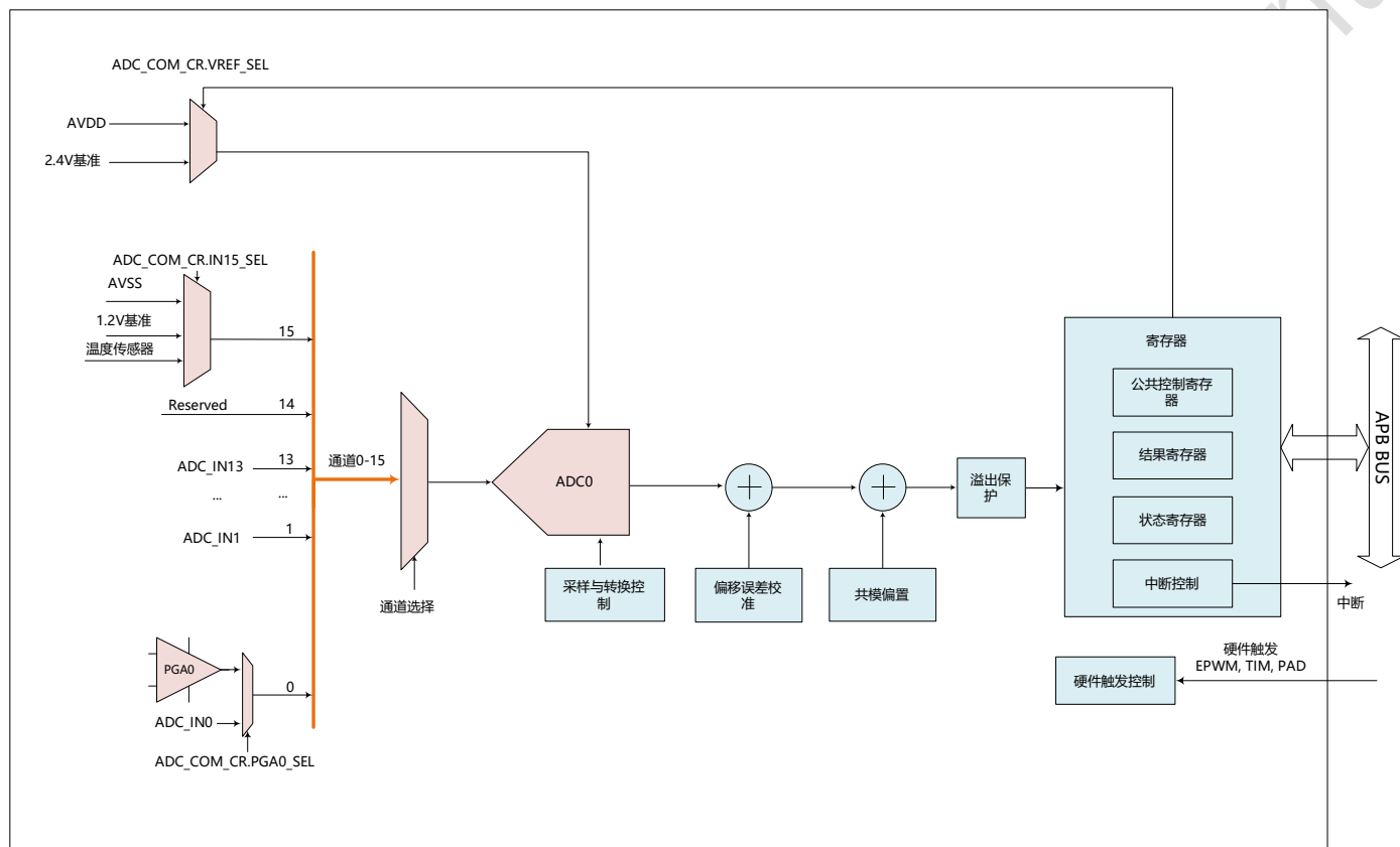
图 19-1 ADC 模块结构框图
